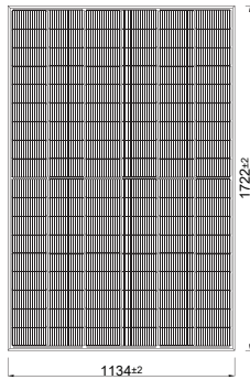
ÖNDEN GÖRÜNÜM
