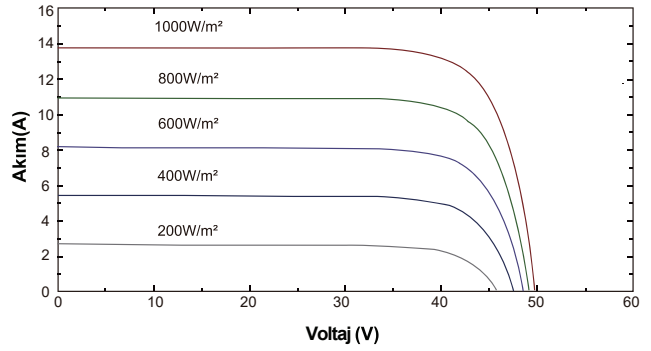
Akım- Voltaj Grafiği (CWT540 -144PM10)
