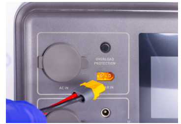
Dönüştürücüyü kullanırken güç kaynağında doğru yuvaya bağlandığından emin olun.
