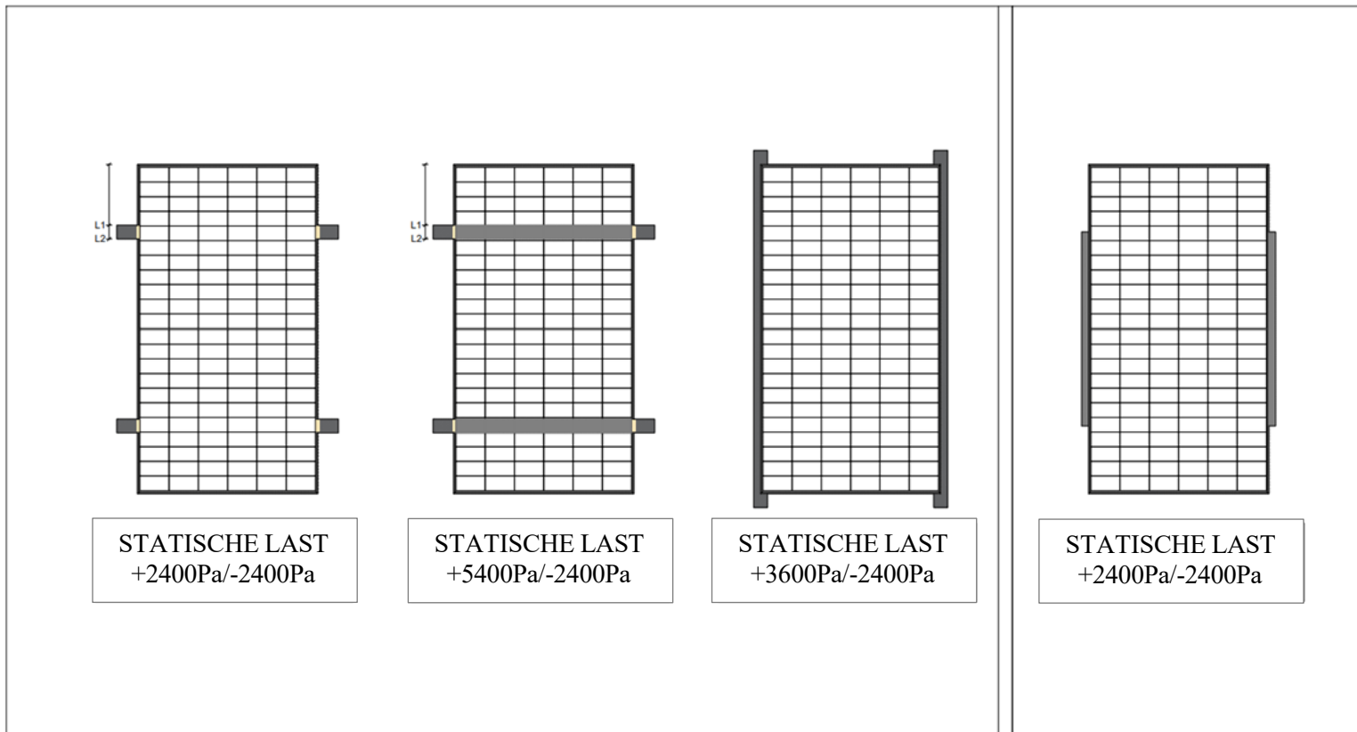
Abbildung 4: Installationsmethoden
