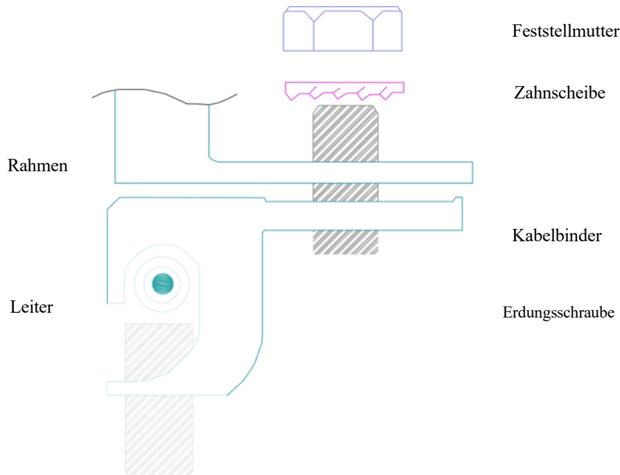
Abbildung 7: Installationsmethoden
