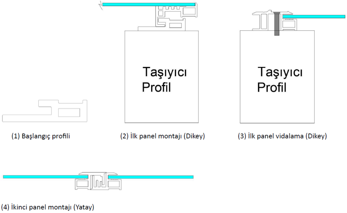
Şekil 2: Montaj Detayları
