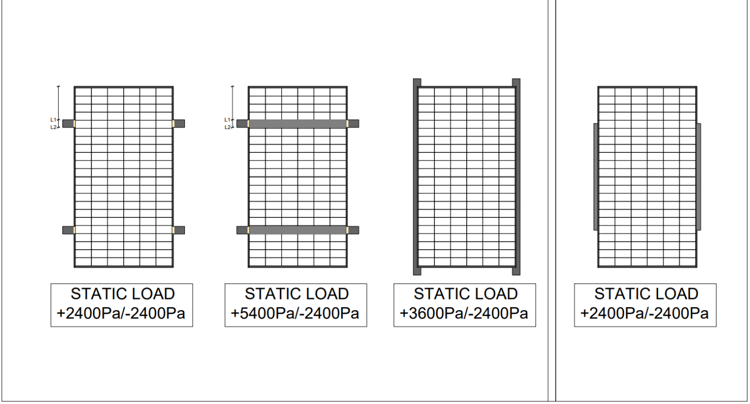
Şekil 4: Kurulum Metodları
