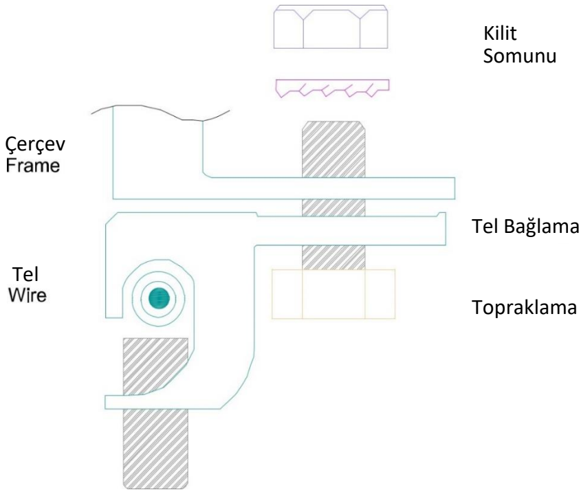
Şekil 8: Montaj Metotları
