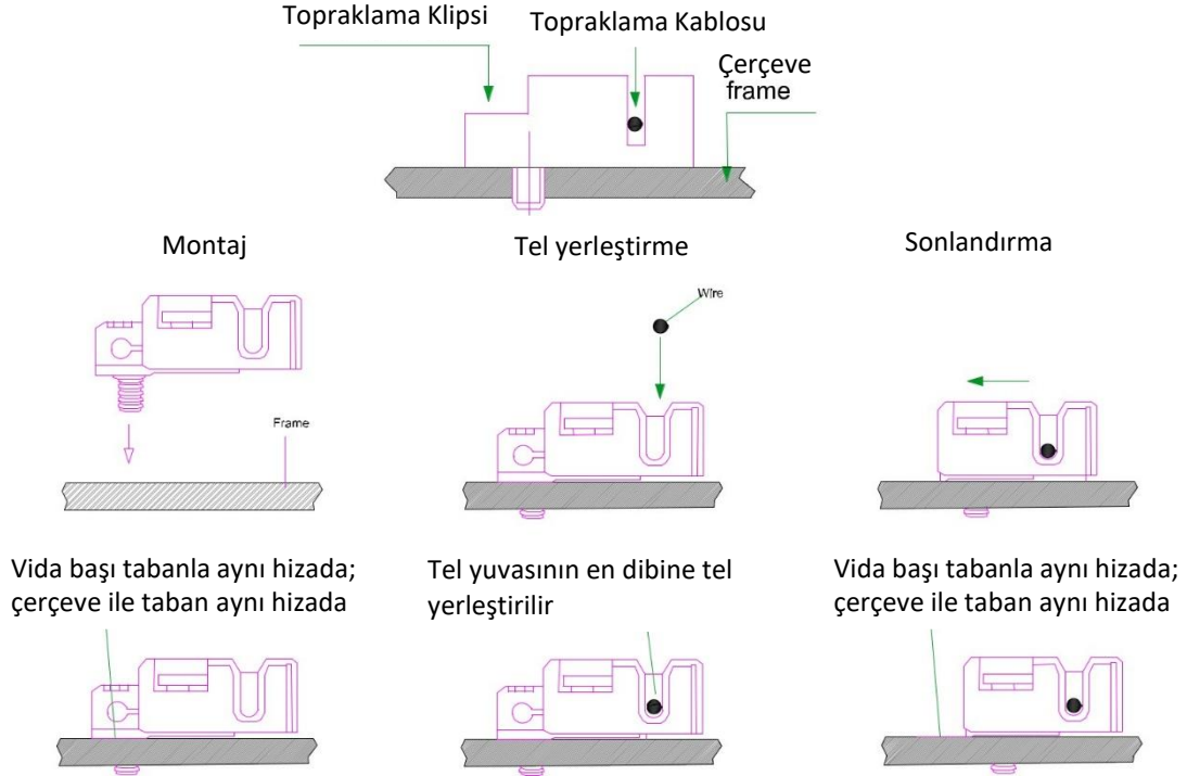
Şekil 7: Topraklama Metotları
