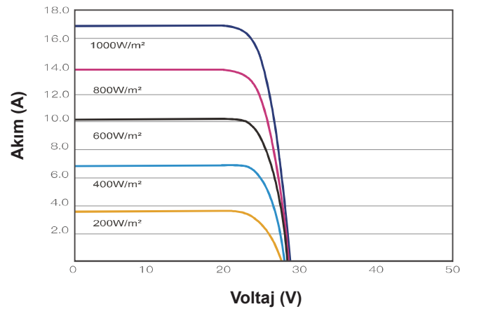
Akım - Voltaj Grafiği ( TT395-80PM12-F )
