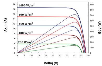
Akım - Voltaj &amp; Güç - Voltaj Grafiği (CWT715-132TNB12)
