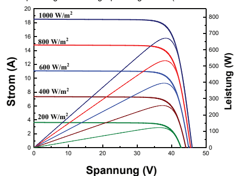
Strom-Spannungs & Leistung-Spannungs Kurve (TT670-132PM12)
