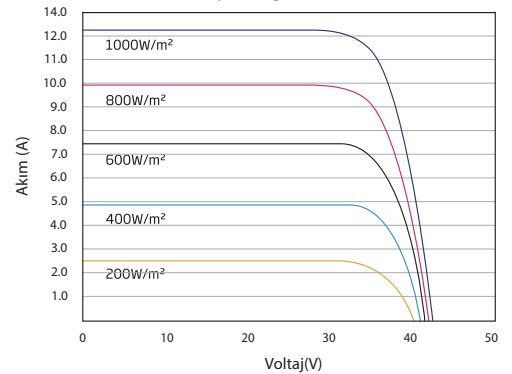
Akım - Voltaj Grafiği (TT400-120TPM12-F)
