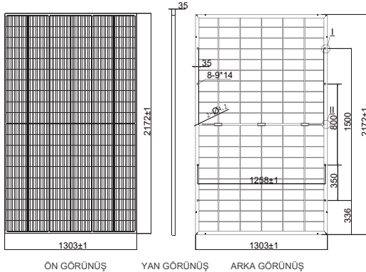
ÖN GÖRÜNÜŞ
