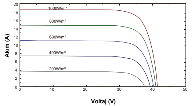
Akım - Voltaj Grafiği (TT600-120PM12)
