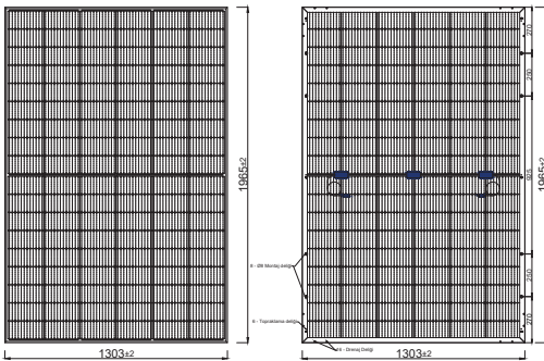
ÖNEN GÖRÜNÜM
