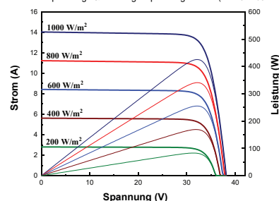
Strom - Spannungs & Leistung - Spannungs Kurve (TT445 - 108TNB10)
