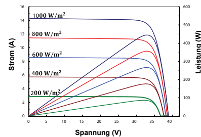
Strom - Spannungs & Leistung - Spannungs Kurve (CWT445 - 108TNB10)
