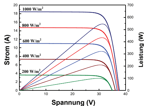
Strom-Spannungs & Leistung-Spannungs Kurve (TT540-108PMFB12)
