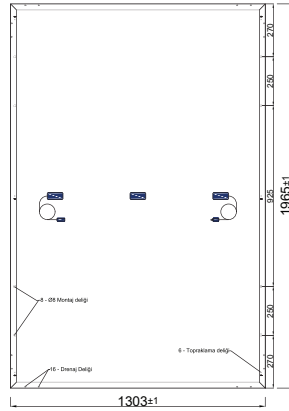
ARKADAN GÖRÜNÜM
