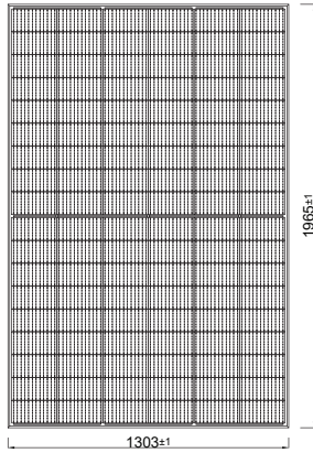
ÖNDEN GÖRÜNÜM
